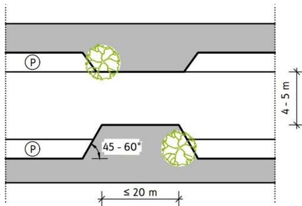
Фиг. 10а. Едностранно локално стеснение
