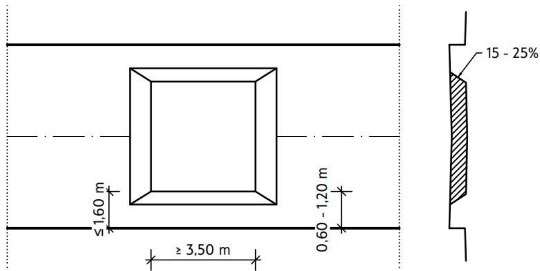
Фиг. 3б. Цяла пътна възглавница на двулентово платно за движение
