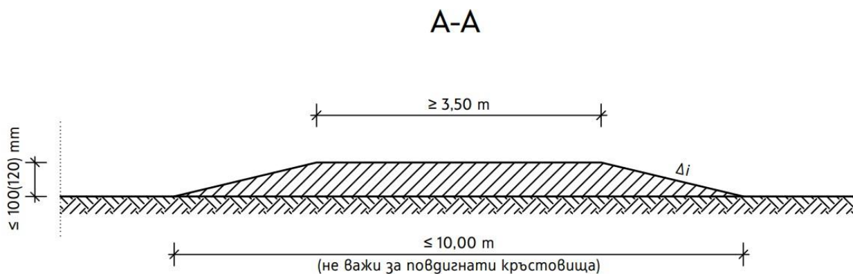
Фиг. 2г. Надлъжен разрез на пътна табла, пътна възглавница и на повдигнато кръстовище
