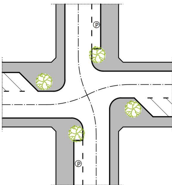
Фиг. 9а. При улици с габарит, по-голям от 12 m и двупосочно движение
