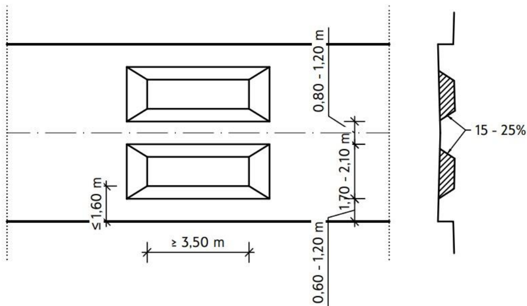
Фиг. 3а. Отделени пътни възглавници на двулентово платно за движение
