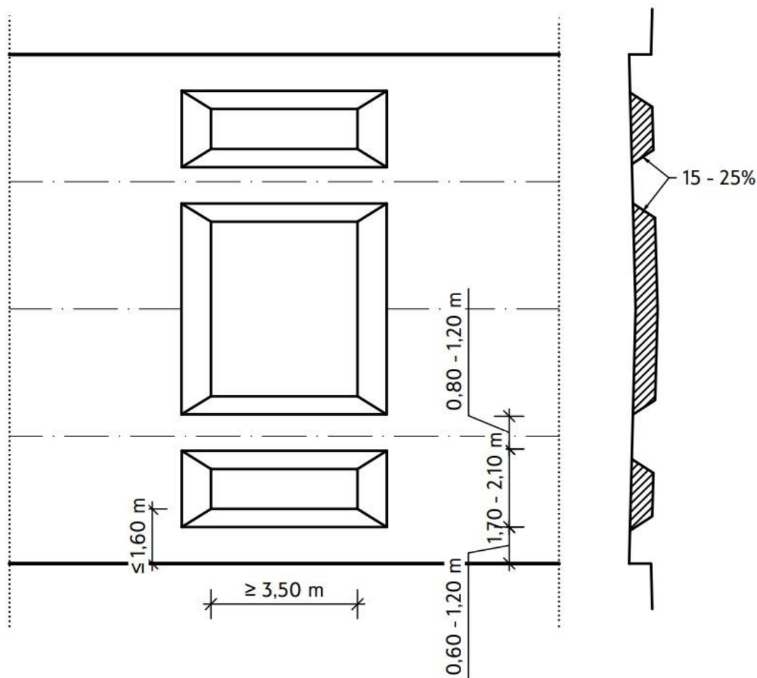
Фиг. 3в. Отделени възглавници на многолентово платно за движение
