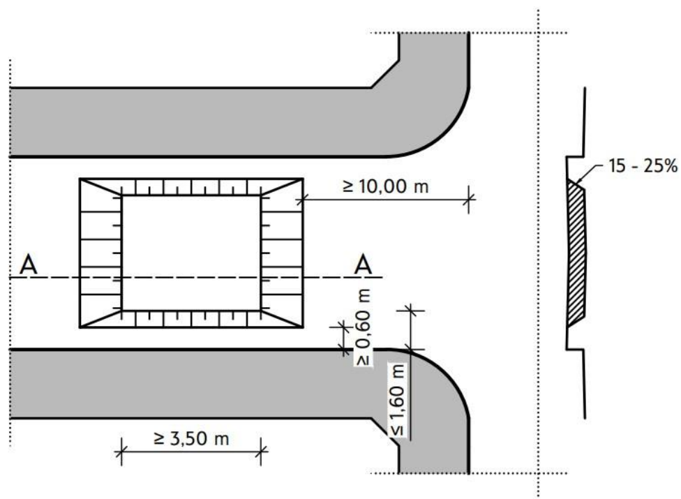
Фиг. 2б. План и напречен разрез на пътна възглавница
