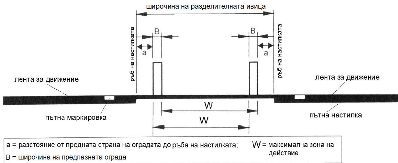
Фигура 17. Едностранна ограничителна система за пътища с разделено действие, разположена до рѐба на настилката
