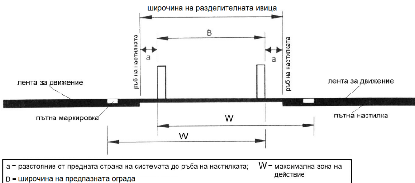
Фигура 18. Едностранна ограничителна система за пътища с общо действие, разположена до рѐба на настилката
