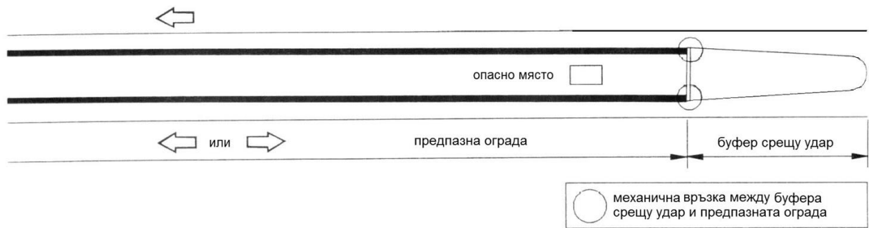
Фигура 20. Ограничителна система изградена двустранно в разделителната ивица от едностранна ограничителна система за пътища с буфер срещу удар за начало
