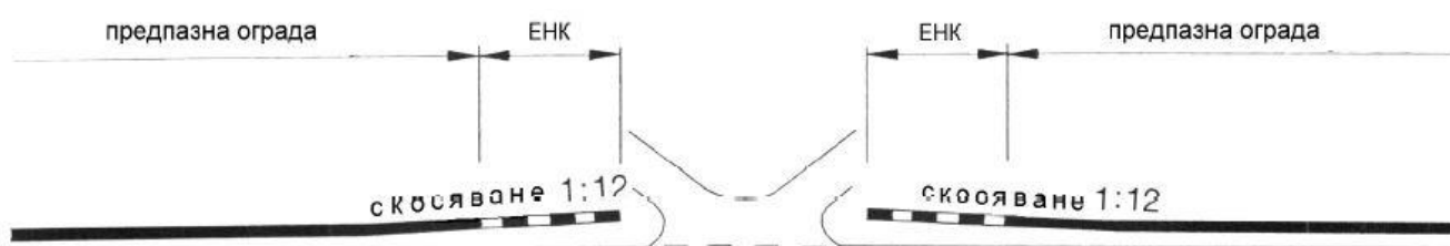
Фигура 9а Прекъсване на ограничителна система за пътища скосена навън 1:12 и с елементи за зануляване
