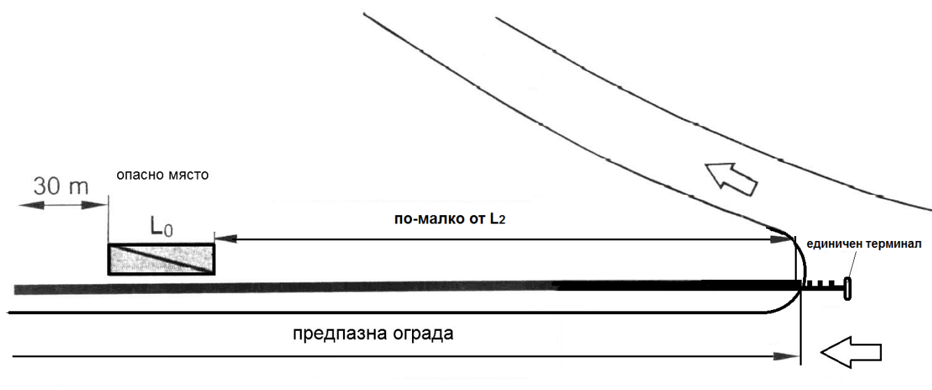
Фигура 11. Ограничителна система за пътища с елементи за начало – единичен терминал при недостатъчно L_2 , включително при разделяне на потоци
