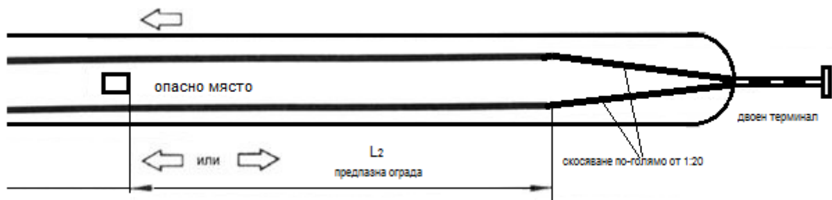
Фигура 22. Ограничителна система изградена двустранно в разделителна ивица от едностранна ограничителна система за пътища с начало двоен терминал
